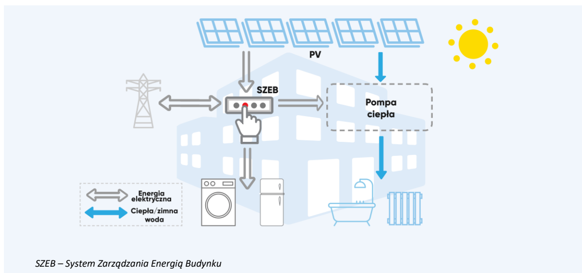
Rys. 7 Konceptcja zintegrowanego systemu energetycznego budynku
